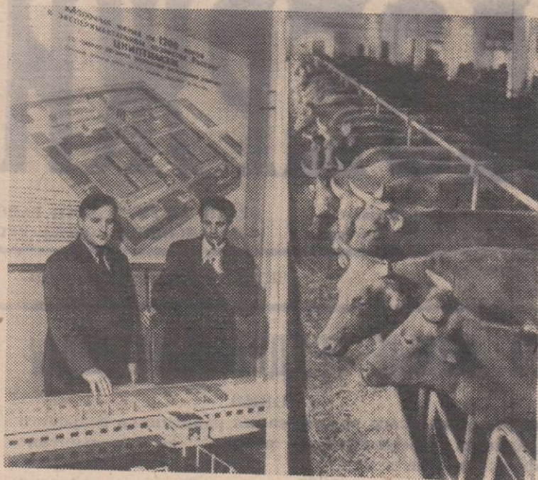
Запорожская область. Специалисты Центрального научно-исследовательского проектно-технологического института механизации и электрификации животноводства Южной зоны СССР разработали сменно-поточную систему обслуживания коров на молочных комплексах промышленного типа.
